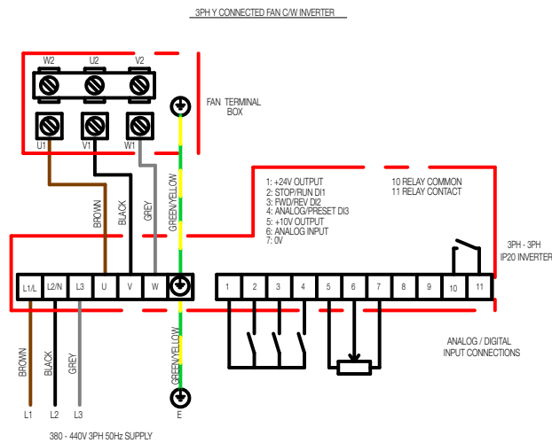
3PH Y CONNECTED FAN C/W INVERTER
