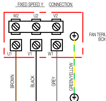
3PH Y CONNECTED FAN C/W INVERTER
