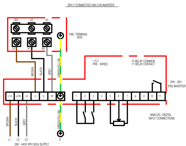
3PH Y CONNECTED FAN C/W INVERTER
